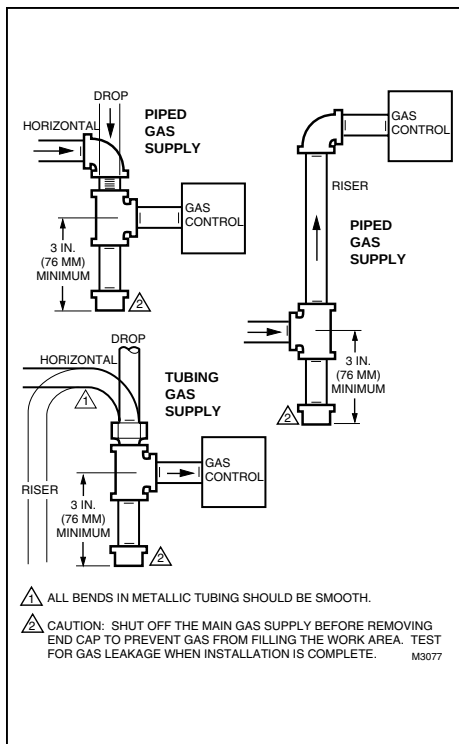
Fig. 1—Install sediment trap.
